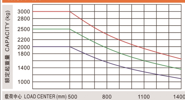
载荷曲线图 Load Curve
